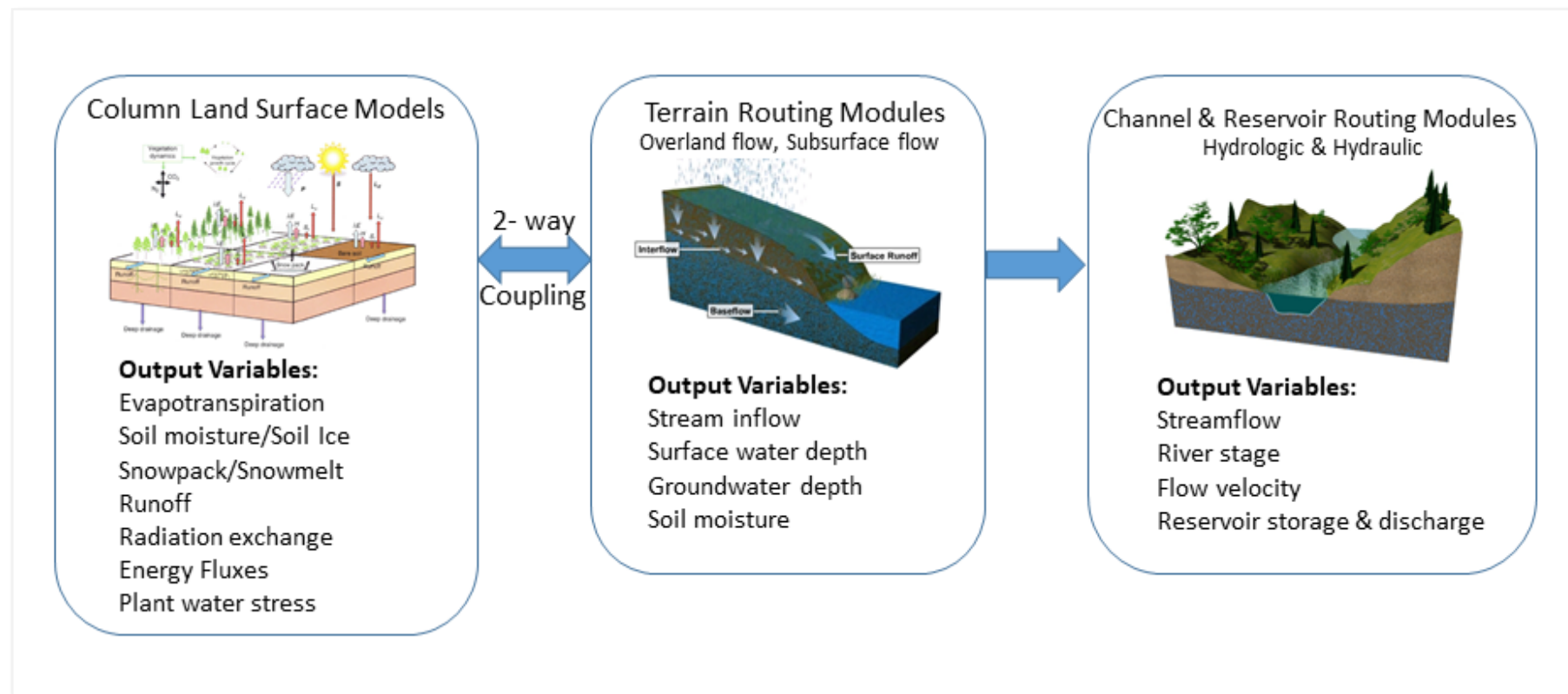
WRF-Hydro 모델의 구성 개념도
