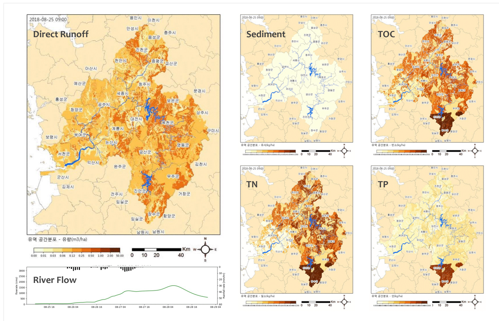
STREAM 모의결과: 유역 내 강우유출 및 오염부하유출의 시공간 분포 (금강 유역, 2018)
