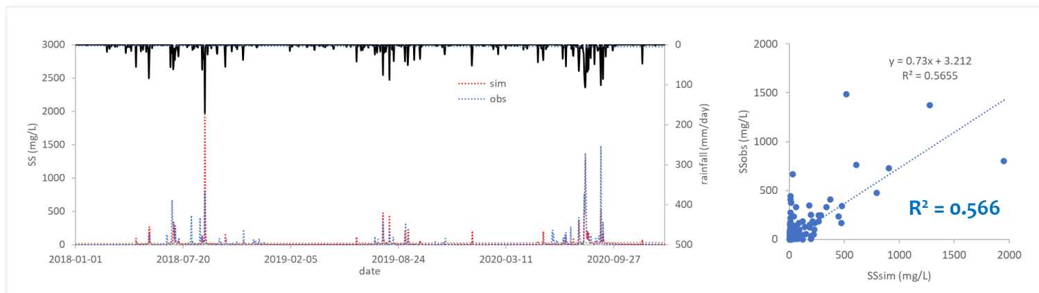
DEWMOST 모의결과: 인북천 유역 말단의 1일 평균 부유사 농도 (2018 - 2020)
