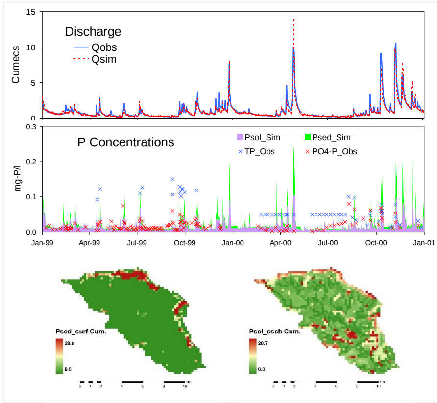
CAMEL 모의결과: 소유역 내 인의 주요오염원 지역 분석 (Tarland Catchment, Scotland, 1999 - 2000)
