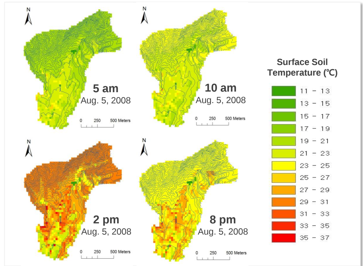
CAMEL 모의결과: 표층 토양온도의 시공간 분포 (경기도 여주군 오계리, 2008)
