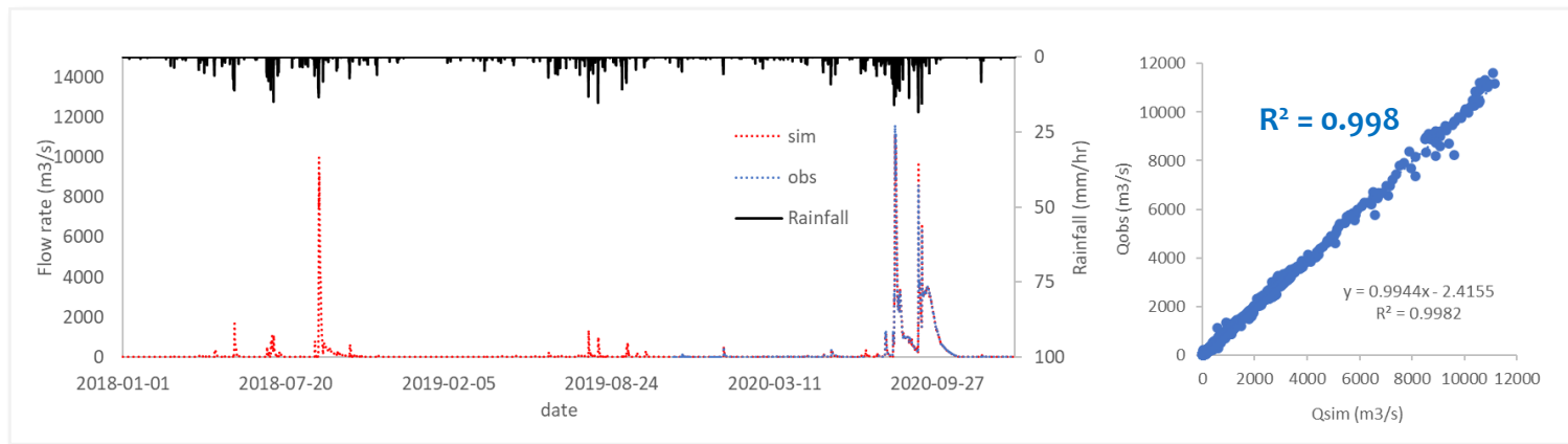
DEWMOST 모의결과: 인북천 유역 말단의 1시간 유량 (2018 - 2020)
